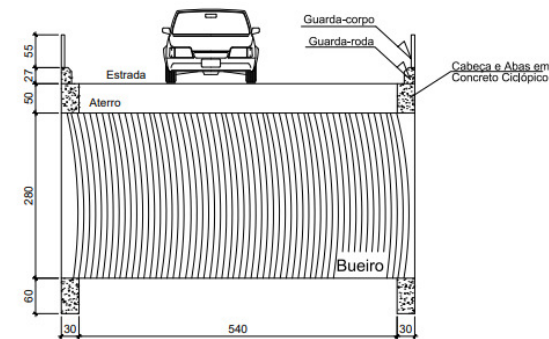
SEÇÃO LONGITUDINAL SEM ESCALA
