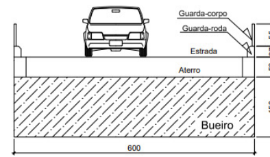
DETALHE DO COMPRIMENTO DO BUEIRO SEM ESCALA
