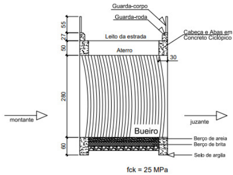
SEÇÃO TRANSVERSAL SEM ESCALA
