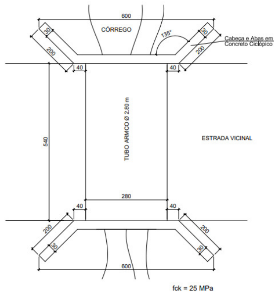
PLANTA BUEIRO ARMCO SEM ESCALA
