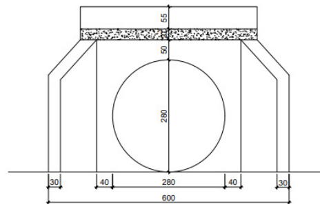
VISTA FRONTAL SEM ESCALA
