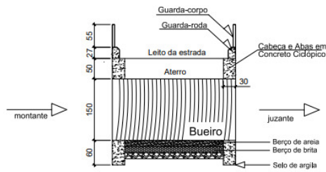
SEÇÃO TRANSVERSAL SEM ESCALA
