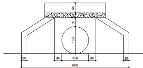
VISTA FRONTAL SEM ESCALA
