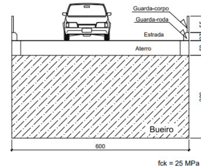
DETALHE DO COMPRIMENTO DO BUEIRO SEM ESCALA
