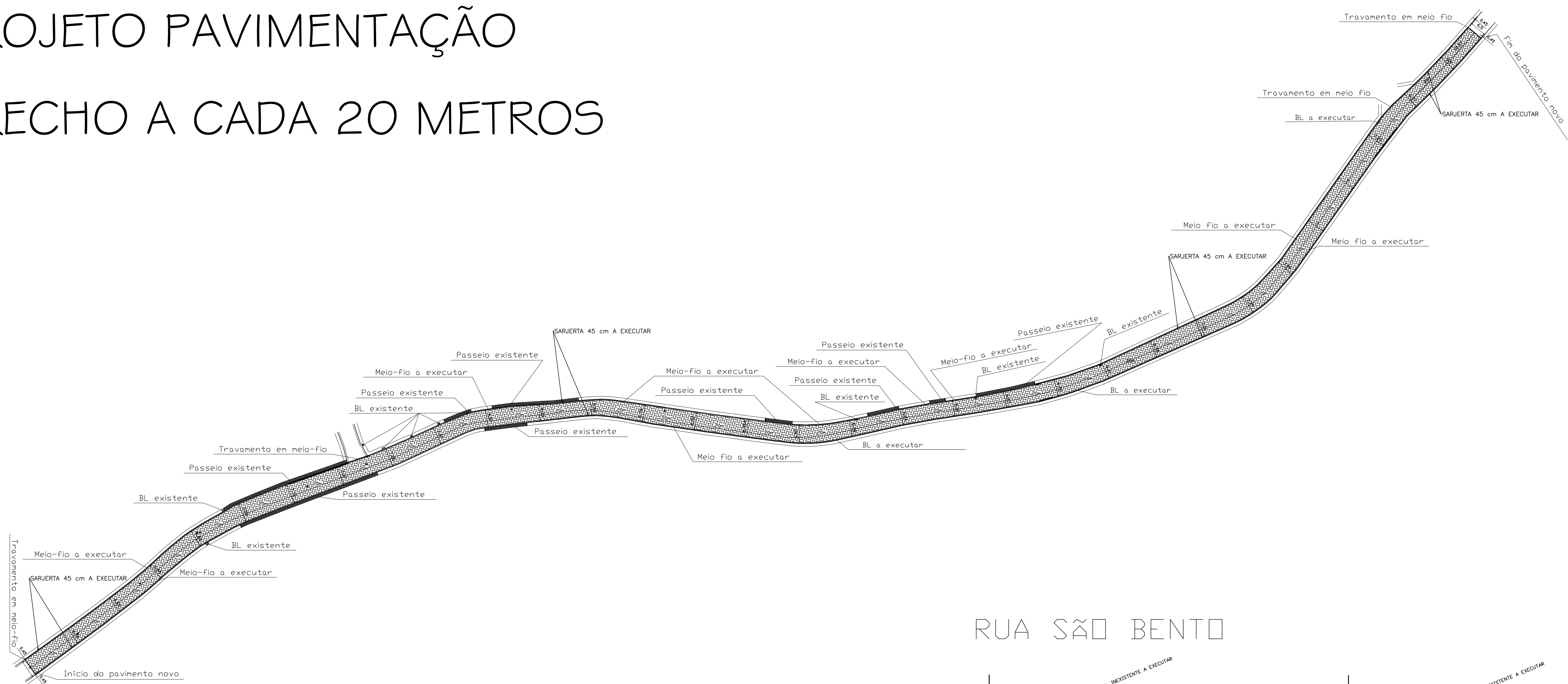
PLANTA TRECHO DA RUA SÃO BENTO
